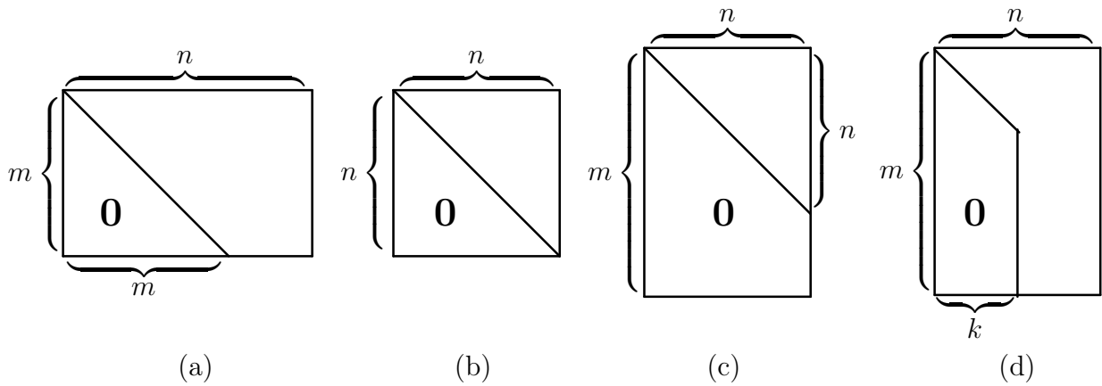
Рис. А.4. Схематическое представление возможных случаев применения теоремы ?? к матрице A(m, n) ; (a) недоопределенная система: k = m - 1 \leq n ; (b) определенная система: k = n - 1, m = n ; (c) переопределенная система: k = n < m ; (d) k < n < m
