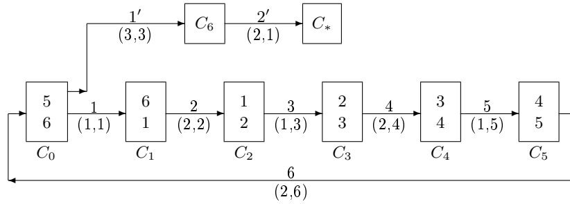
Рис. 6.2.2. Зацикливание и выход из цикла в задаче И. М. Л. Биля
