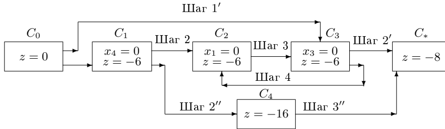
Рис. 6.2.1. Граф решения с возможным заикливанием: C_0 — исходное состояние; C_* — оптимальное состояние; C_1, C_2, C_3 — состояния в одной из трех совпадающих вершин, в которых одна из базисных переменных (соответственно, x_4, x_1, x_3 ) равна нулю; C_4 — за пределами допустимой области.
